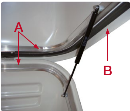
Mit Aluminiumrahmen (A) und wasserfesten Dichtungen (B) verstärkt
